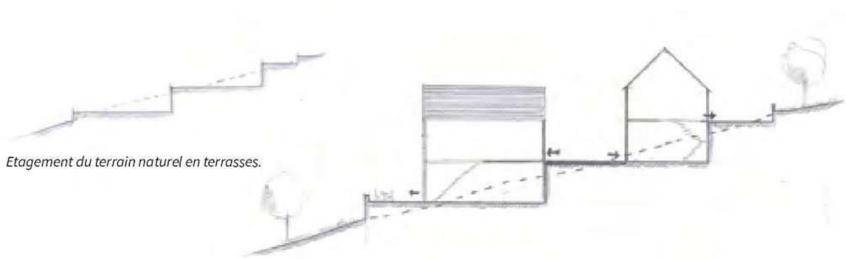
Implantation des maisons en profitant du dénivelé, gestion d'accès haut et bas.
