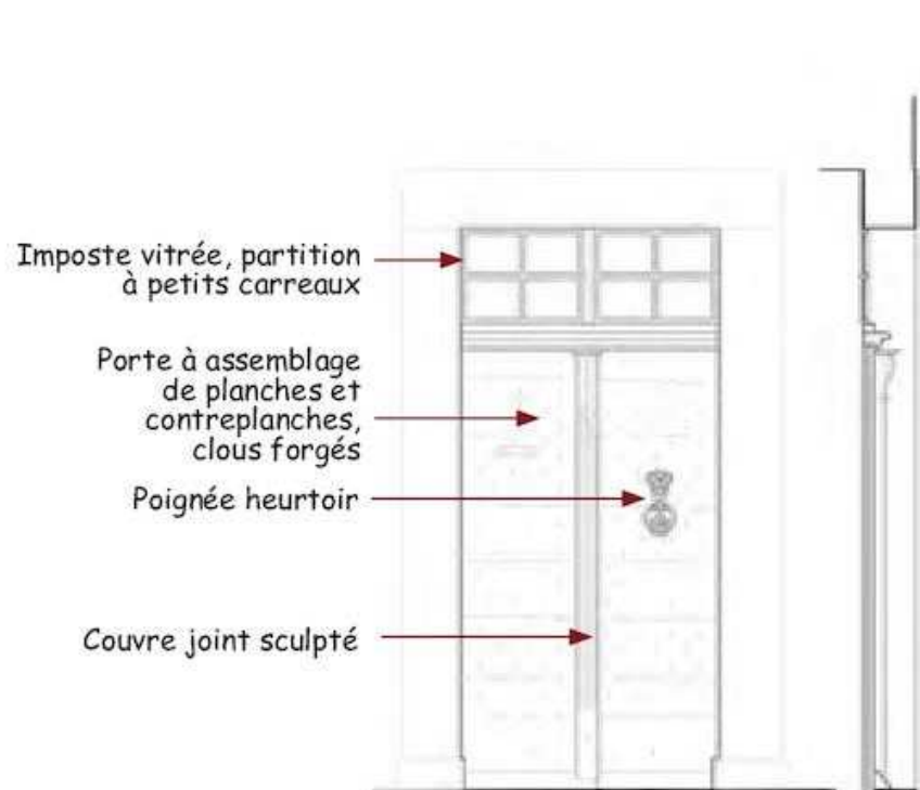
Porte type XVIII e siècle, vantail double, imposte vitrée, menuiserie à planches et contre planches, cloutage.
