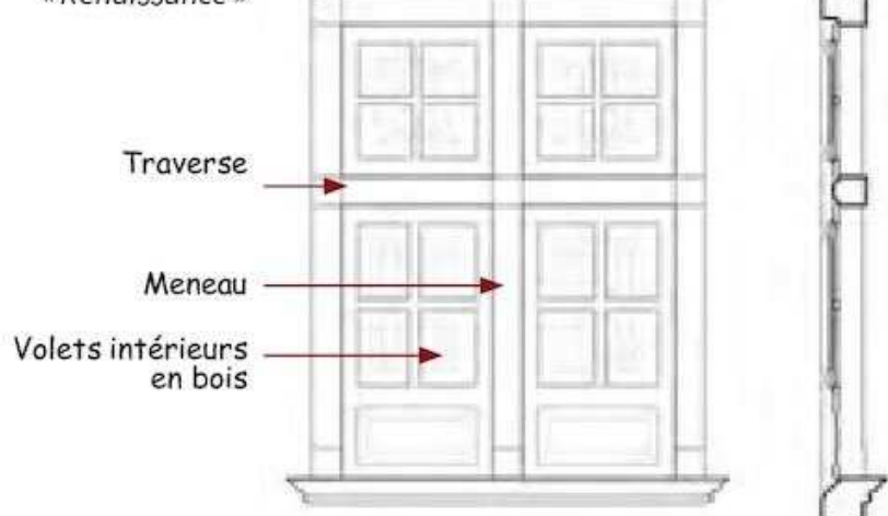
Croisée de type « Renaissance »
