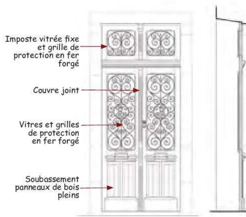
Porte type XX e siècle, vantail double, menuiserie et vitrage, imposte, grilles de protection en ferronnerie.
