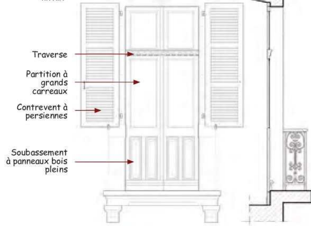
Porte fenêtre fin XIX e
